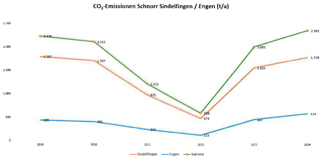
Entwicklung der aus Energieträgern resultierenden CO 2 -Emissionen
